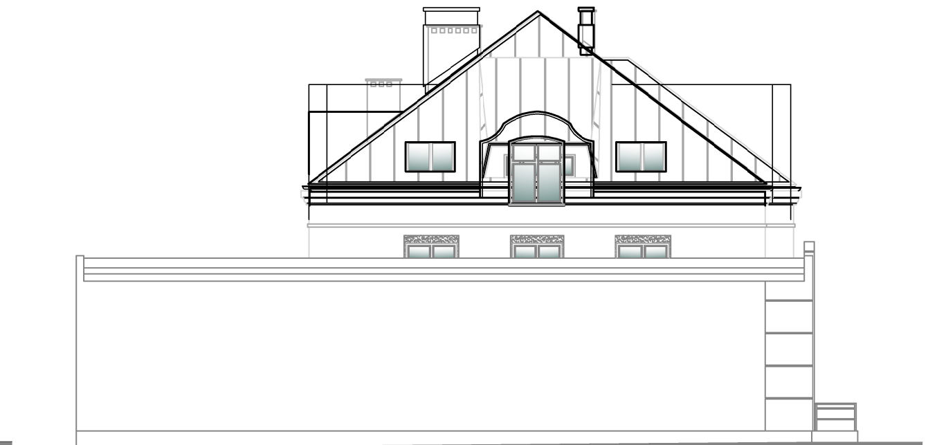
ELEWACJA WSCHODNIA-BOCZNA
